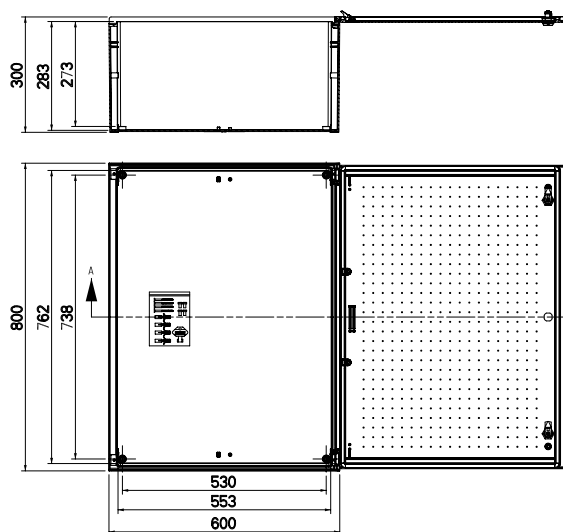
Montageplatte 86M800
